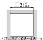
■パネルカット寸法
